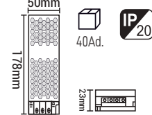
30A SLIM KASA ADAPTÖR MX-3032
