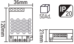
16.5A SLIM KASA ADAPTÖR MX-3028
