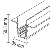
TRIMLESS L DÖNÜŞ APARATI MX-4540 Tavan
