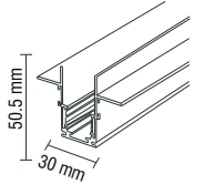
TRIMLESS L DÖNÜŞ APARATI MX-4541 Duvar
