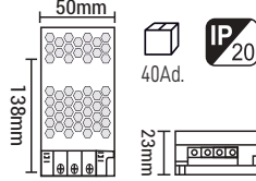
20A SLIM KASA ADAPTÖR MX-3030
